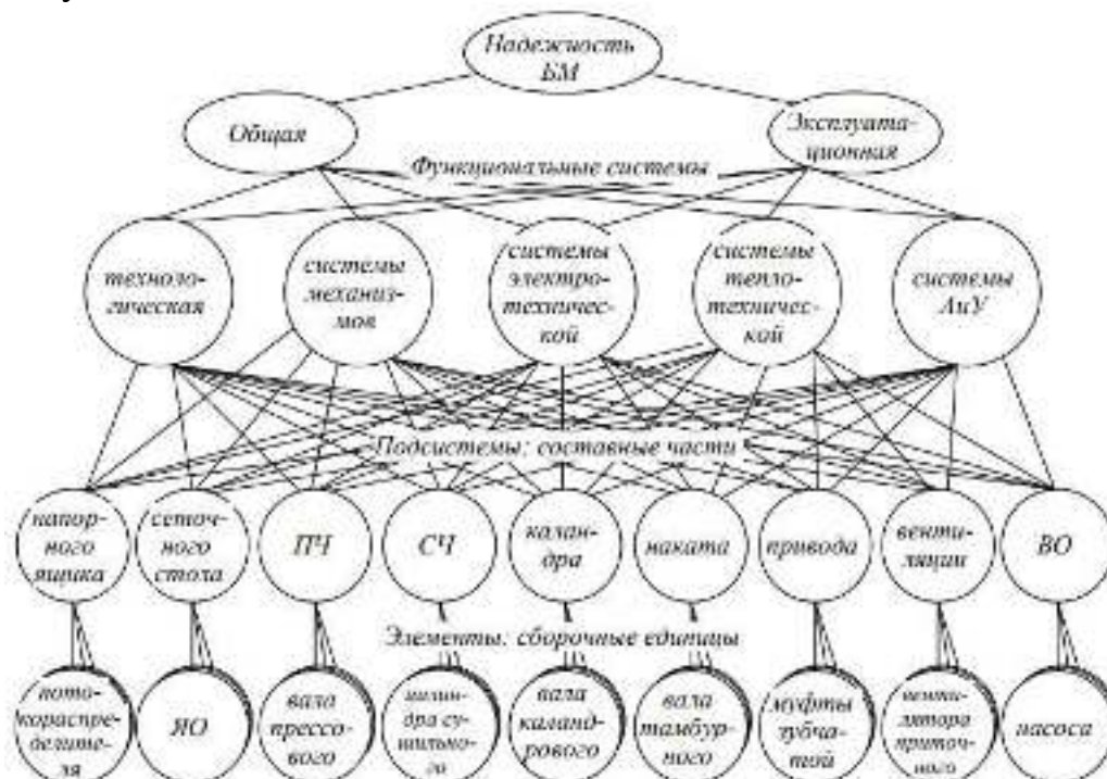
Рис. 1 – Иерархическая структура надежности БМ: системы АиУ – системы автоматизации и управления; ВО – вспомогательного оборудования; СЧ – сушильной части; ПЧ – прессовой части; ЯО – ящика отсасывающего
