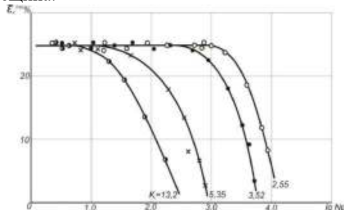
Рис. 3. Кривые измерения e_i (%) от числа циклов до разрушения.
