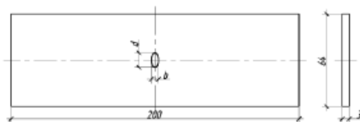
Рис. 1. Чертеж образца
