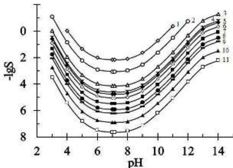
Рис. 1. Зависимости молярной растворимости S (моль/л) твёрдых оксидов и гидроксидов алюминия от величины pH водной среды при 25 0 С. 1- Al 2 O 3 (аморфный), 2- γ-Al 2 O 3 , 3- Al(OH) 3 (аморфный), 4- δ-Al 2 O 3 , 5- κ-Al 2 O 3 , 6- β-Al(OH) 3 (нордстрандит), 7- α-Al 2 O 3 (корунд), 8- α-Al(OH) 3 (байерит), 9- γ-AlO(OH) (бемит), 10- γ-Al(OH) 3 (гиббсит), 11- α-AlO(OH) (диаспор)
