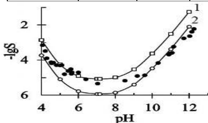
Рис. 2. Сравнение рассчитанных в настоящей работе кривых равновесной молярной растворимости S (моль/л) \beta-Al(OH)_3 (1) и \alpha-Al(OH)_3 (2) с экспериментальными данными (черные точки) работы [3] для смеси этих модификаций при 25 0 С.
