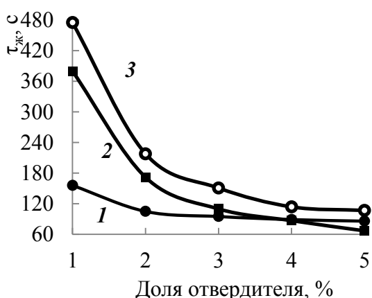
Рис 1. Изменение времени желатинизации КФС с разными отвердителями: 1 – связующее с хлоридом аммония; 2 – связующее с МО-2СБ; 3 – связующее с МО-2Б
