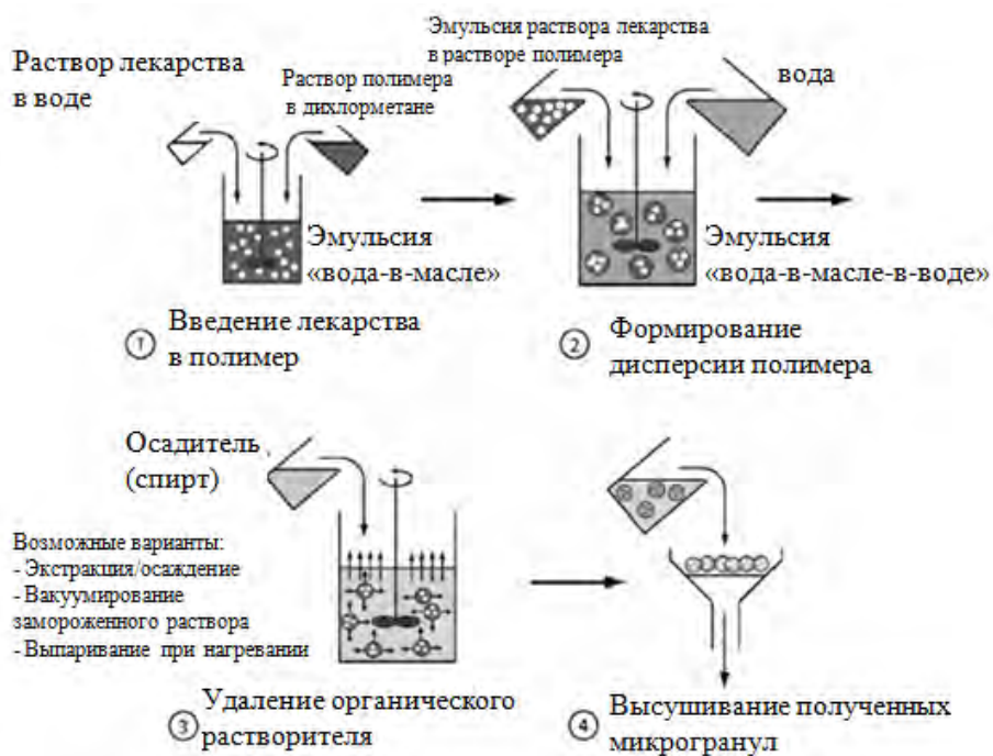
Рис. 3. Укрупненное схематическое представление методики получения микрокапсул методом испарения легколетучего растворителя
