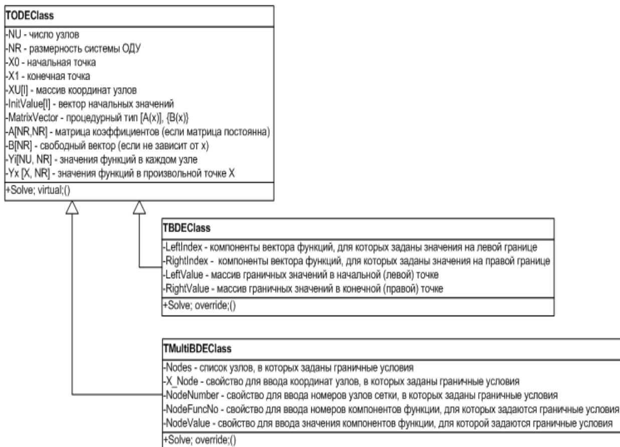
Рис. 1. Иерархия классов
