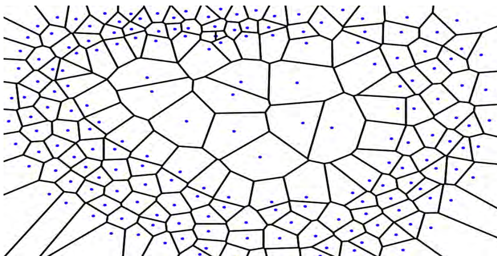
Рис. 2. Многоугольники Вороного
